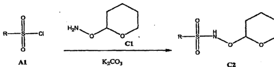
Esquema C. Síntesis general de N -(tetrahidro-piran-2-iloxi)sulfonamidas intermedias.
