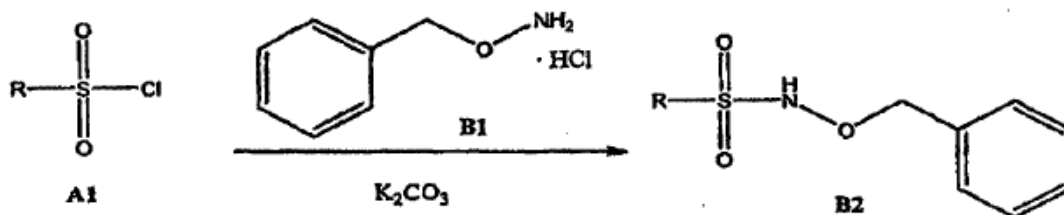
Esquema B. Síntesis general de N -benciloxisulfonamidas intermedias.
