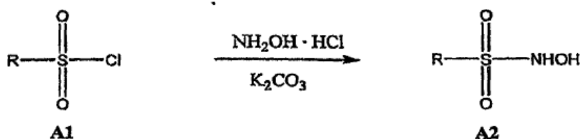
Esquema A. Síntesis general de N -hidroxisulfonamidas.
