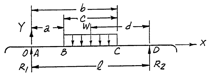
Fig-15A
