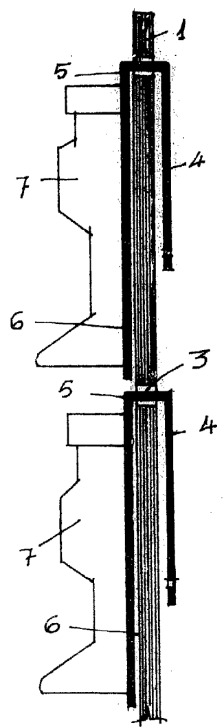
SECCION A-A
