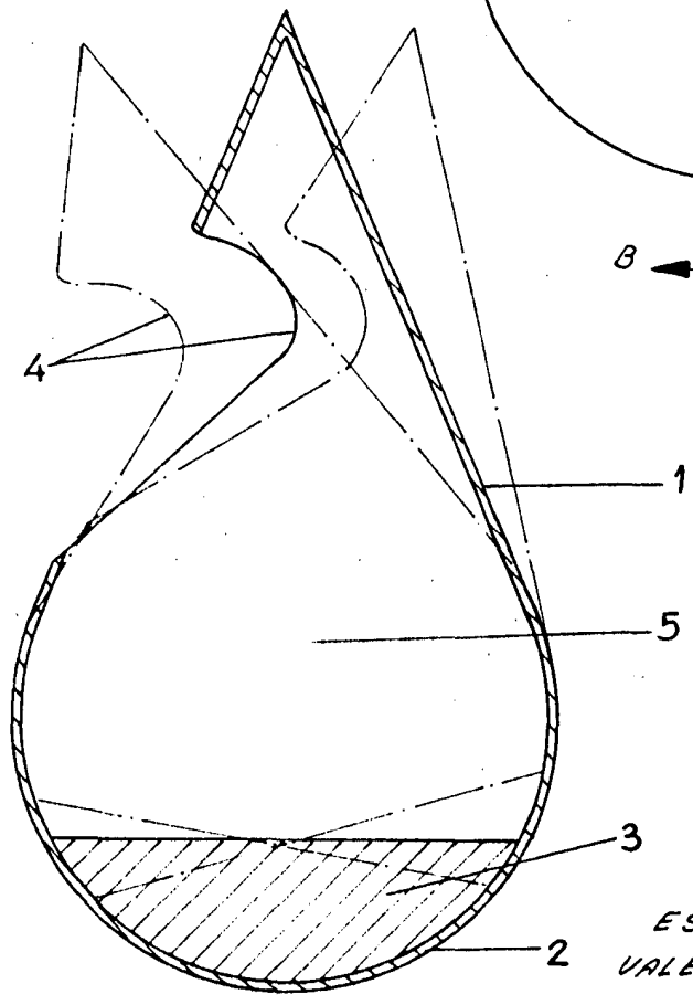
FIG. 2 SECCION A-B
