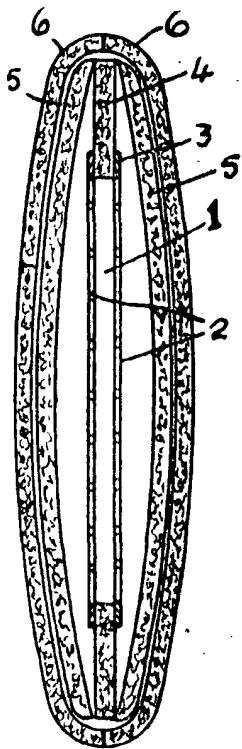
FIG. 2 SECCION A-B
