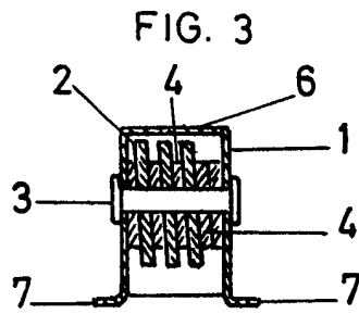
sección A-B
