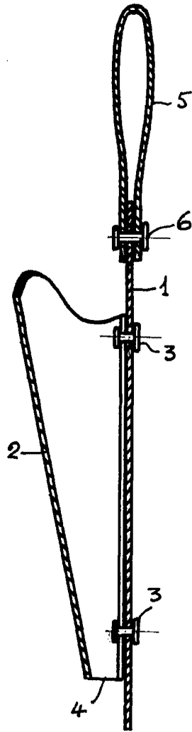
Sección A-B
