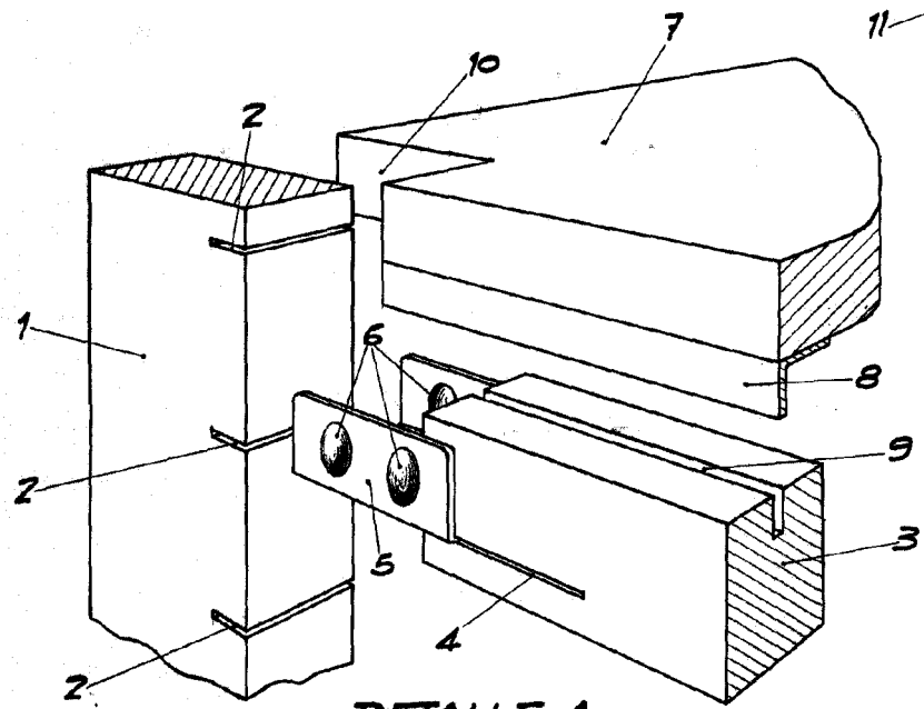
DETALLE-A FIG. 2
